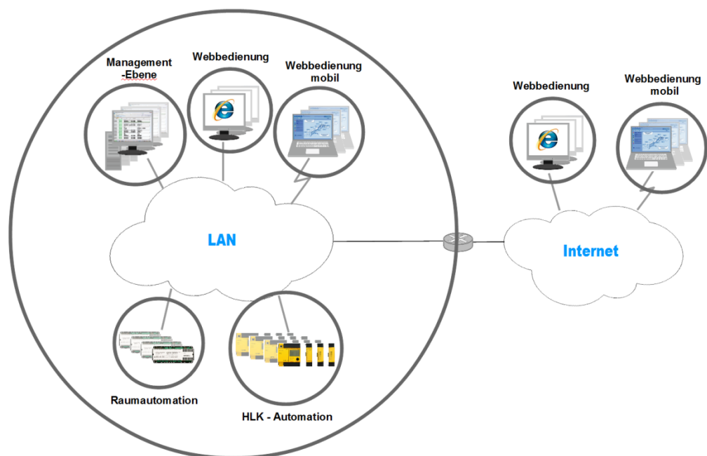
Fig. 1 : Domaines et réseaux du système de GTB
